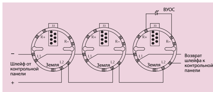
Рис.1 Схема соединений - XP95/Discovery монтажная база
