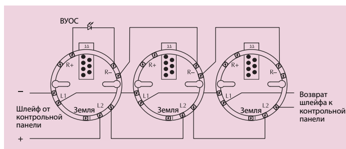
Рис.2 Схема соединений нескольких XP95/Discovery извещателей с общим светодиодом ВУОС
